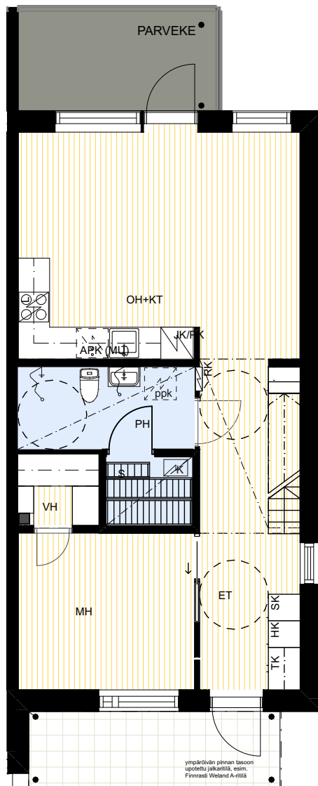
1.kerros
