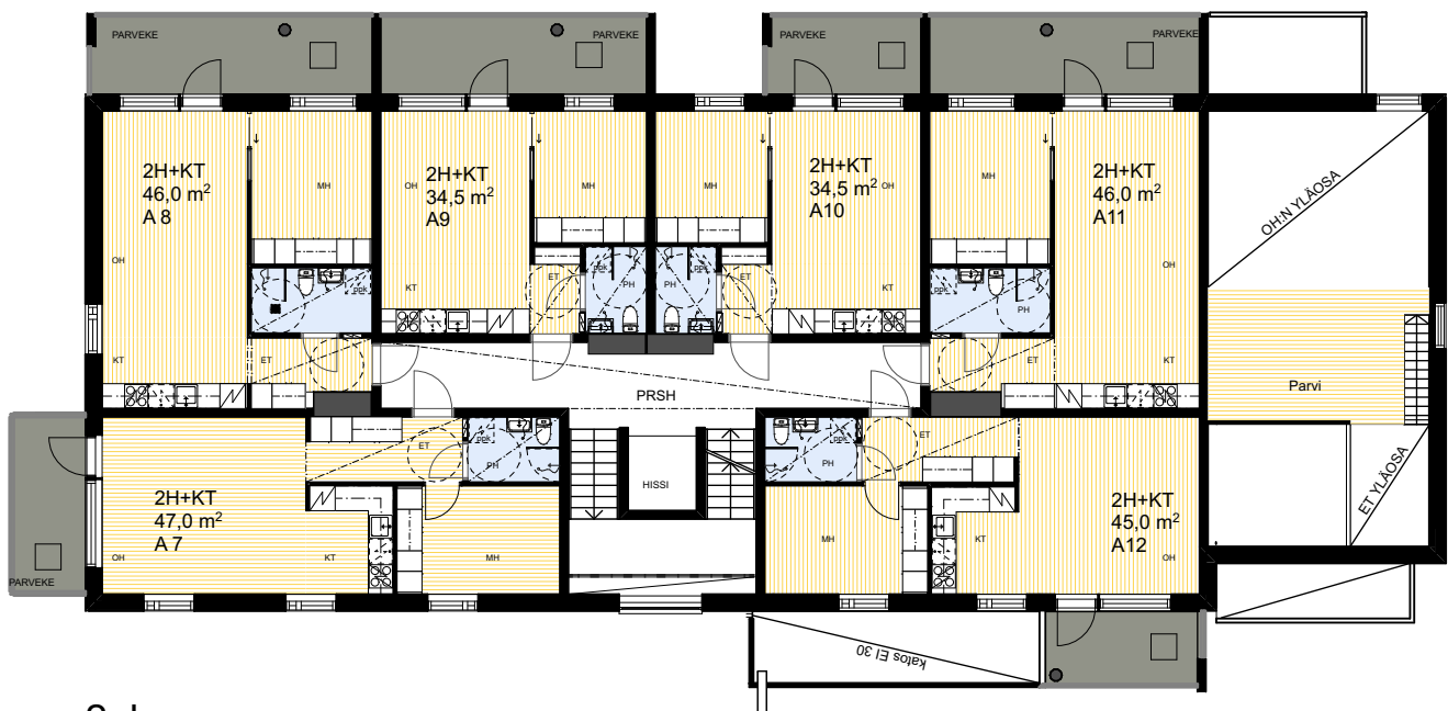
2. kerros
