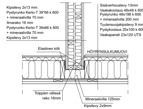
HUONEISTOJEN VÄLISEN SEINÄN LIITTYMINEN ULKOSEINÄÄN 1:20
