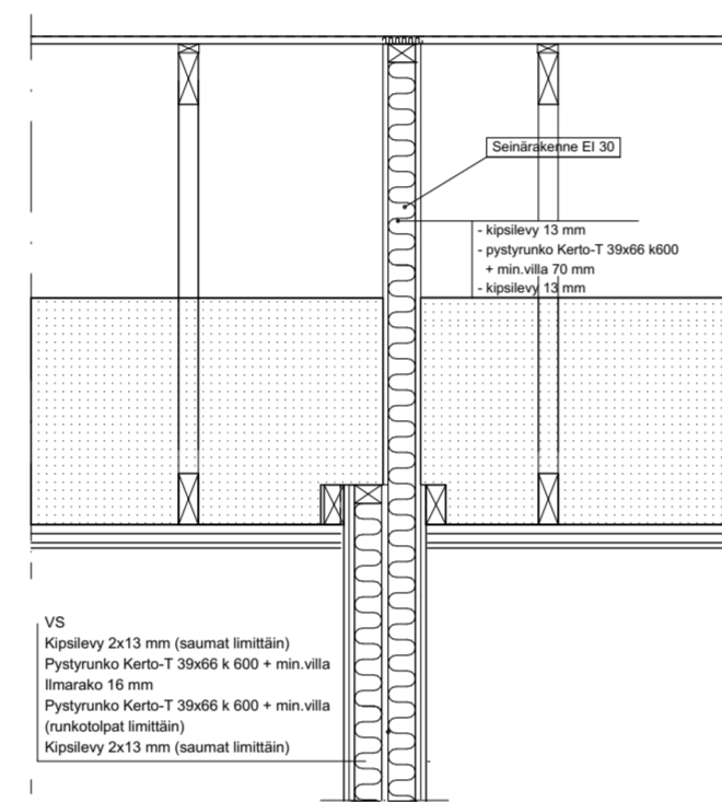
HUONEISTOJEN VÄLINEN SEINÄ 1:20
